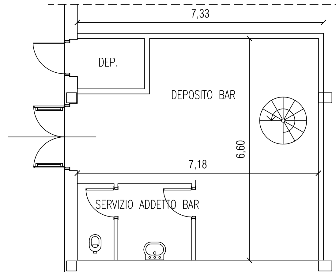
PIANO SEMINTERRATO – BAR (locali di servizio)
