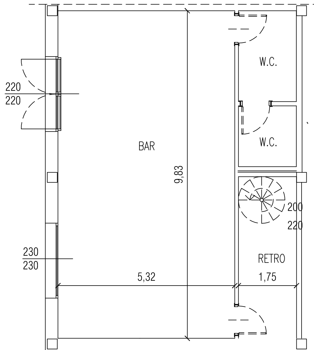
PIANO RIALZATO – BAR
