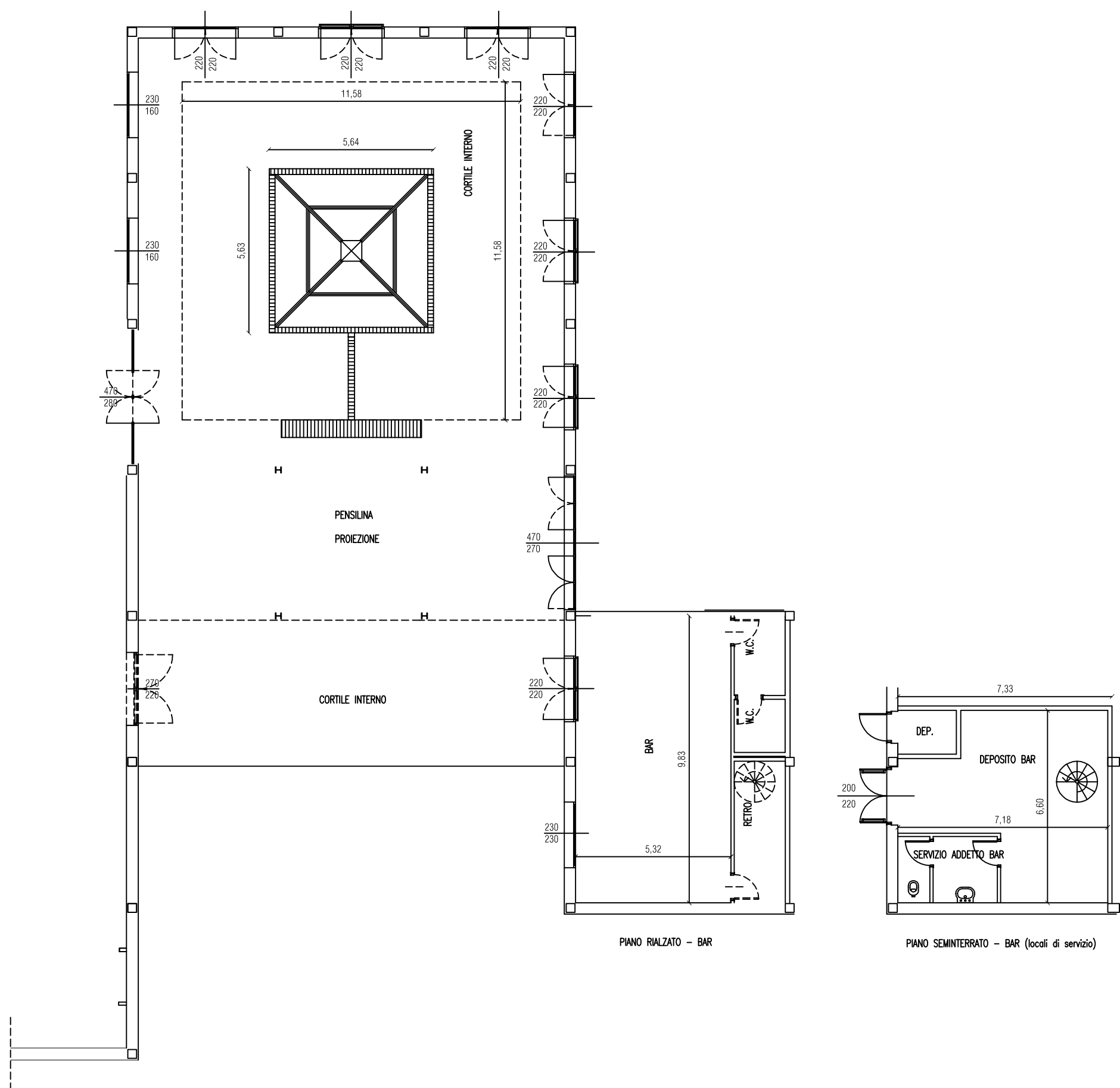
STABILE COMUNALE DI VIA VALVASSORI PERONI 56 Planimetria Piano Seminterrato – BAR (locali di servizio) Planimetria Piano Rialzato – BAR
