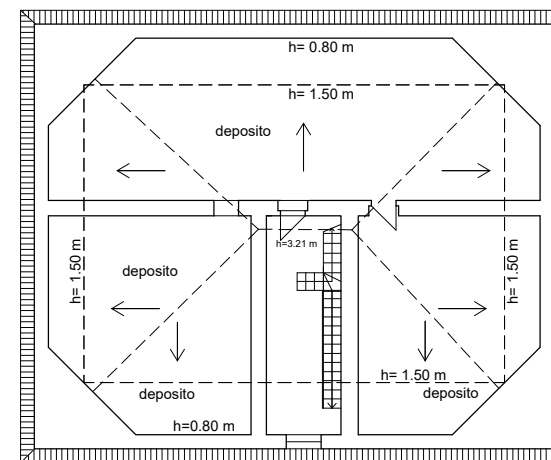
Piano Secondo (fabbr. A)
