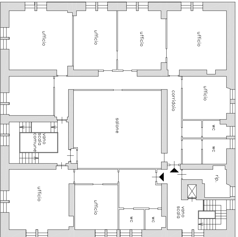
Piano Primo
